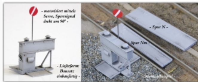
Zub-345.2: Gleiswaage, Typ Filisur, 1 Stück, 3D-Druck, einbaufertig lackiert, für N- und Nm-Gleis, Klett-Modellbau
