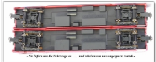
KT-110.3: Umspurung von Kato-Panoramaausgängen aus dem BEX-Set von 9mm auf 6,5mm, Preis pro Wagen
