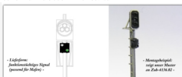
Zub-4136.28: Abfahrtsbefehlssignal (BPAS), funktionsfähig, 1 Stück, Montage am Signalmast (Mafen)
