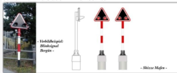
Zub-3832.01: Bahnübergang-Wechselblinksignal, funktionsfähig, 2 Stück, inkl. Steuerung (Hersteller Mafen)
